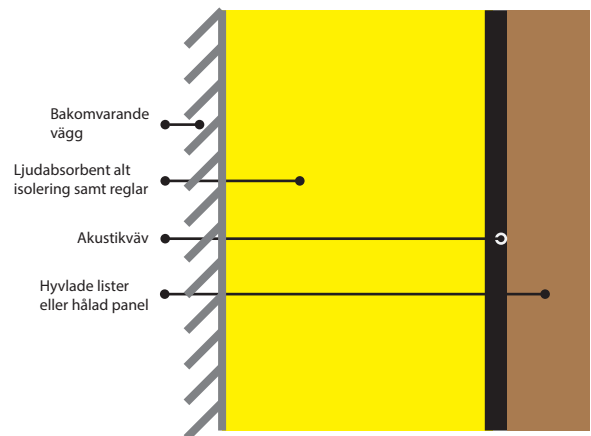
Genomskäring av ljudabsorberande vägg
