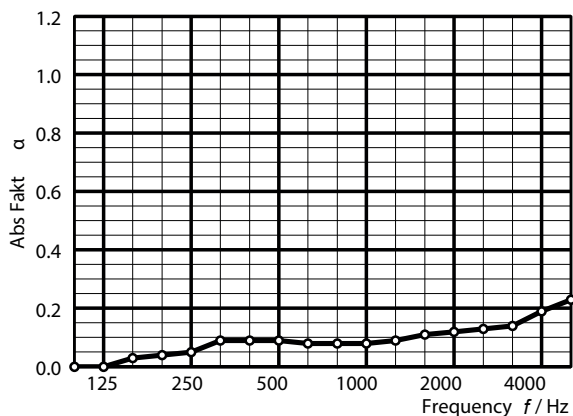
Ljudabsorberingskurva
